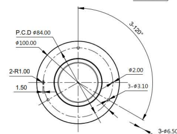
【 Flange 尺寸示意圖】
