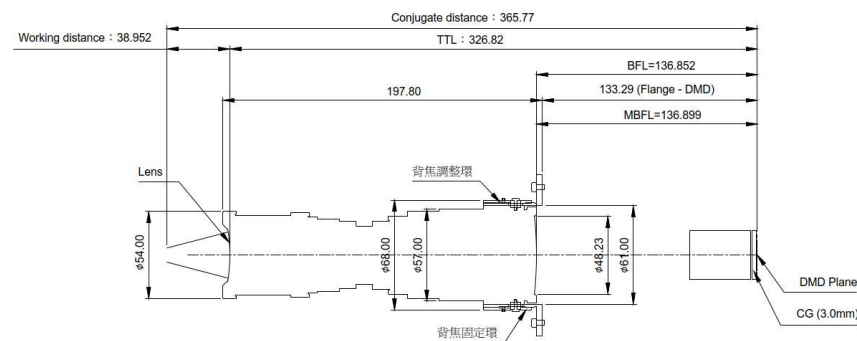
【 Flange 尺寸示意圖】
