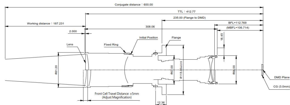
【 Flange Dimension 】
